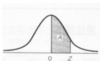
常態分布表
