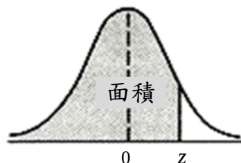
常態曲線下之面積
