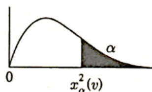
卡方分配右尾機率值之臨界點
