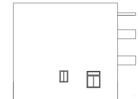
北向立面圖
