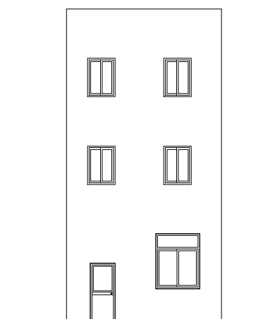
東向立面圖
