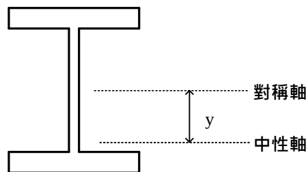
圖 1 H400\times400\times16\times32 中性軸位置示意圖
