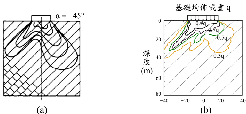
圖二 一組規則節理岩盤上方興建建物之壓力分布傳播
