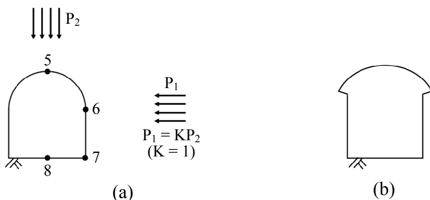
圖一 馬蹄形隧道與傘狀斷面隧道
