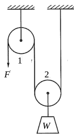
(a)單槽滑車
