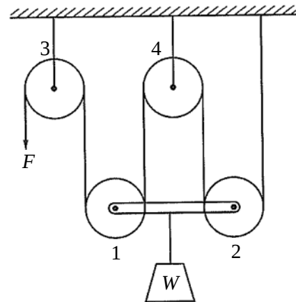
(b)起重用滑車
