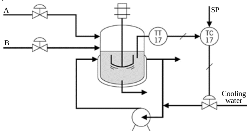
圖2 溫度控制的反應器
