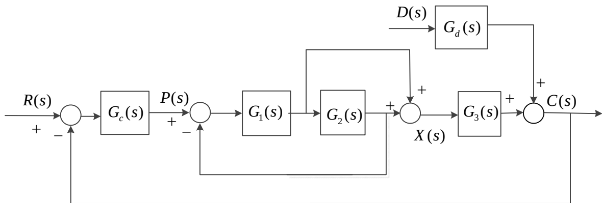
圖1 平行-反饋控制系統
