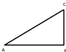
直角三角形 ABC 示意圖
