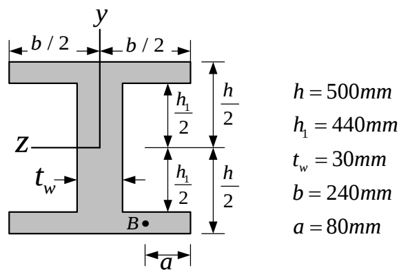
圖四 (b)：梁之截面
