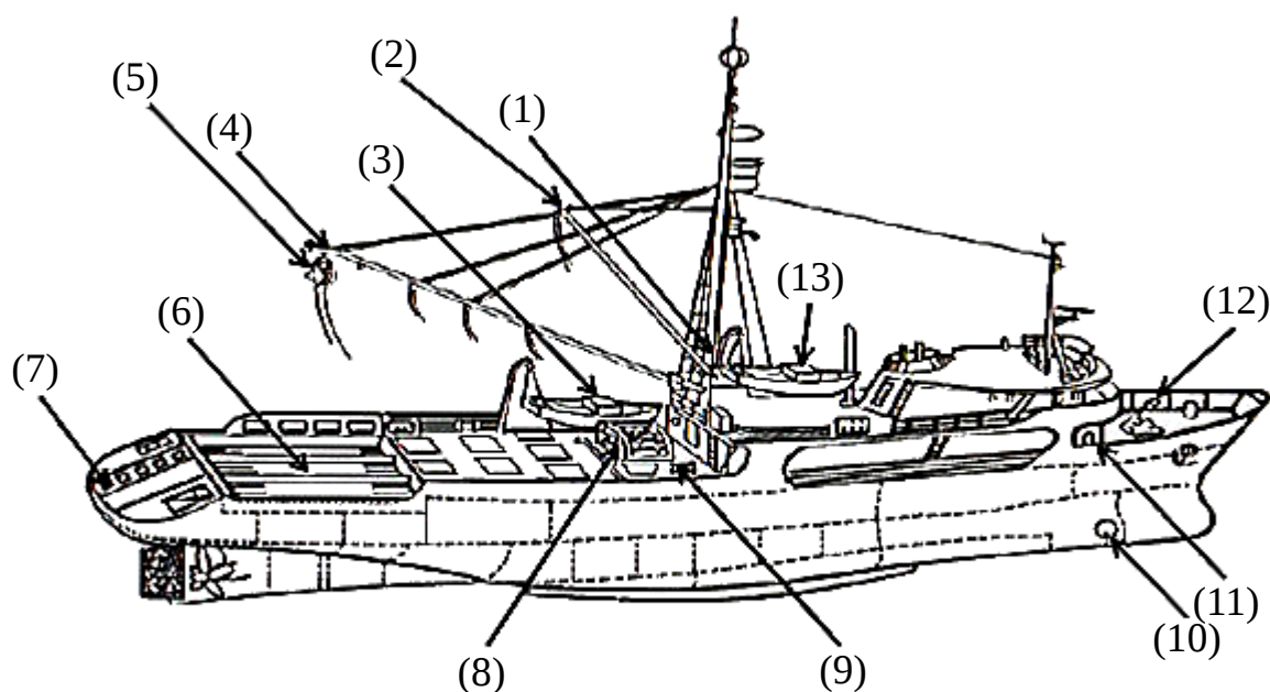
鰹鮪圍網船的漁撈設施配置
