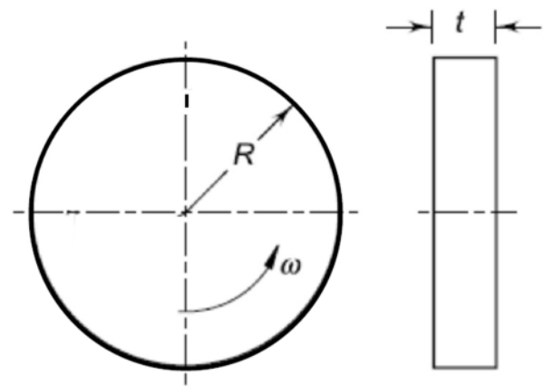
圖三：簡化的圓盤式飛輪
