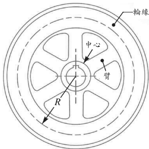
圖二：飛輪
