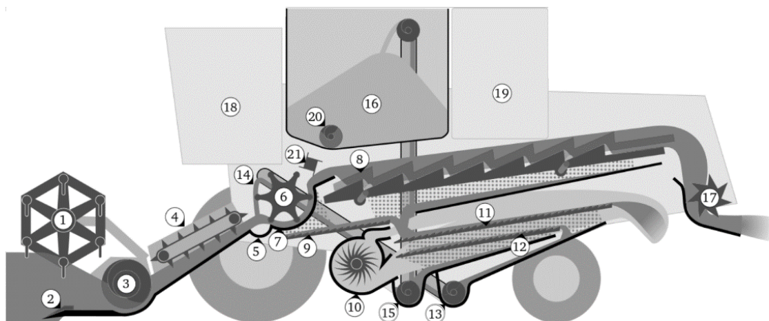
圖一：聯合收穫機示意圖
