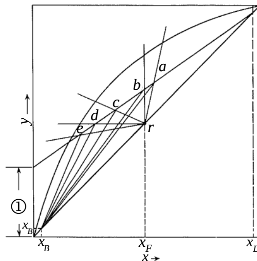
圖三 McCabe-Thiele圖
