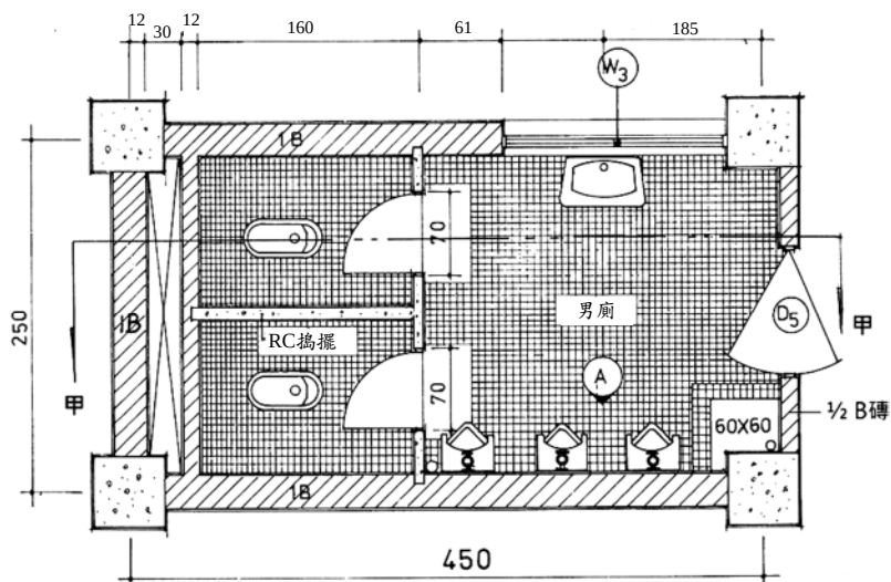
男廁所平面圖
