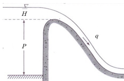
圖2 溢洪道示意圖
