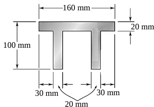
n-n 截面尺寸
