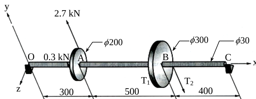
等角速度轉動的軸及滑輪 (尺寸單位為 mm)
