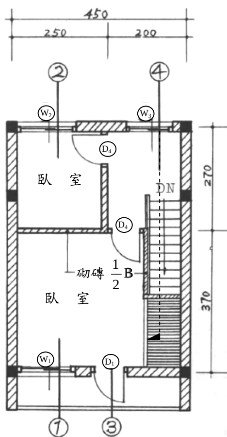
二層平面圖
