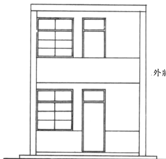
正立面圖
