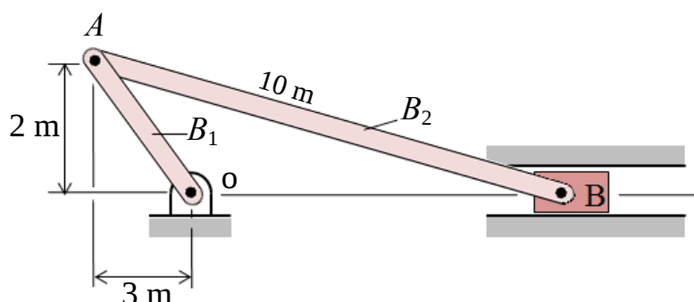
圖三 連桿與滑塊的示意圖 (尺寸未等比例標示)
