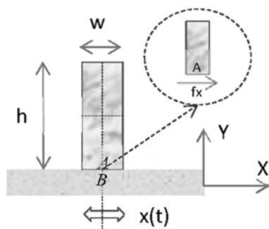
(a) x 方向可運動平台上之矩形梁
