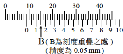
(a) 游標卡尺量測讀數
