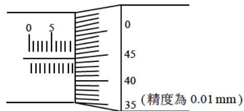
(b) 分厘卡量測讀數
