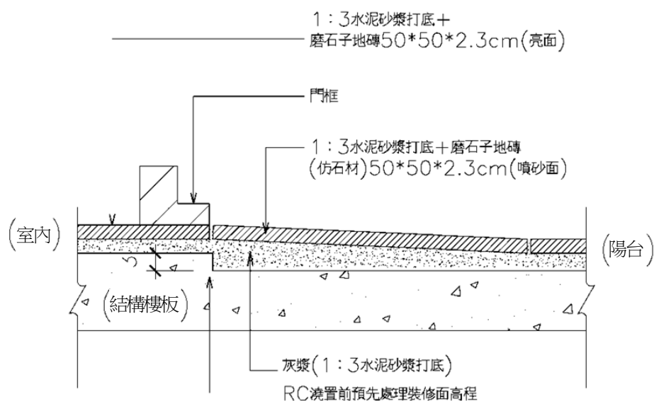
室內及走廊地坪剖面圖（單位：公分）
