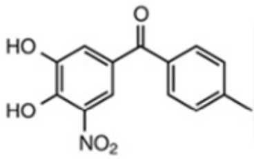
Tolcapone
