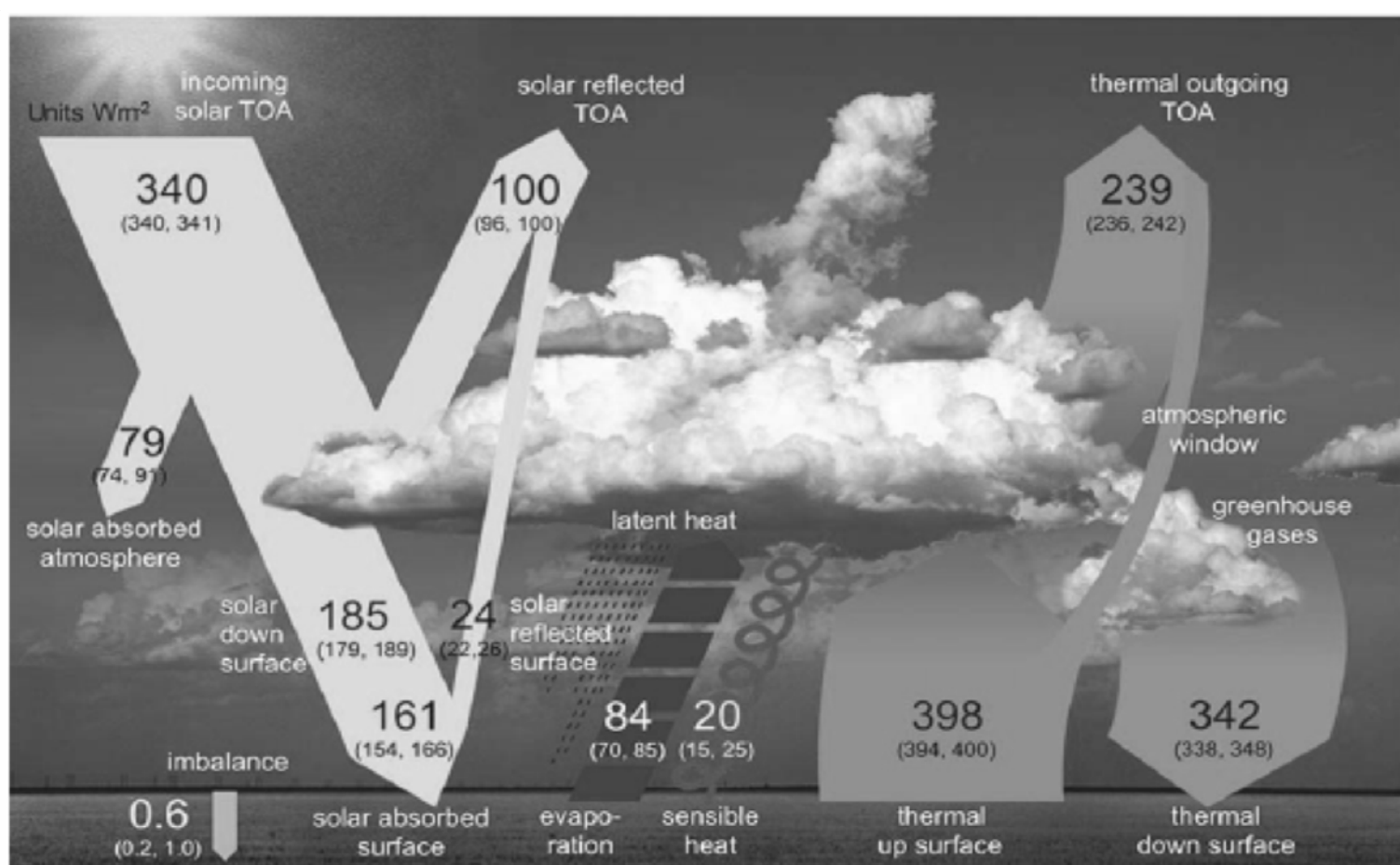
圖一：全球平均能量的收支圖，單位： \text{W/m}^2 。(IPCC AR5, 2013)
