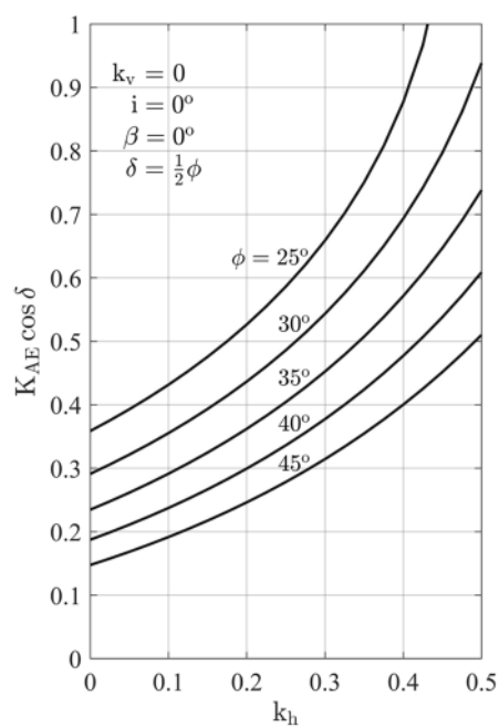
Mononobe - Okabe之主動土壓力係數
