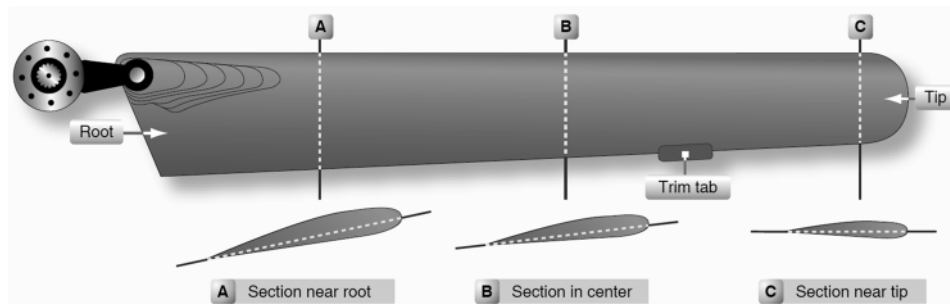
圖 1、主旋翼於不同位置之傾角
