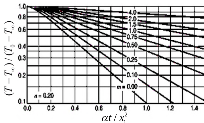
非穩態下平板的內部不同時間與位置的溫度變化圖
