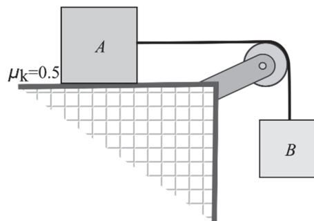
圖(七)
