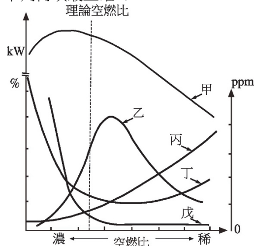
圖(十一)
