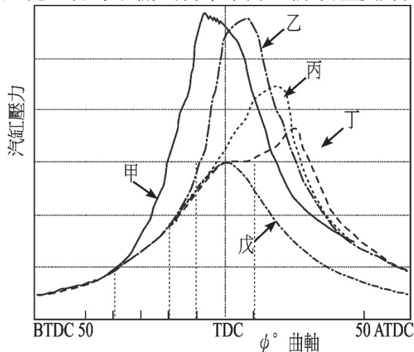
圖(十四)
