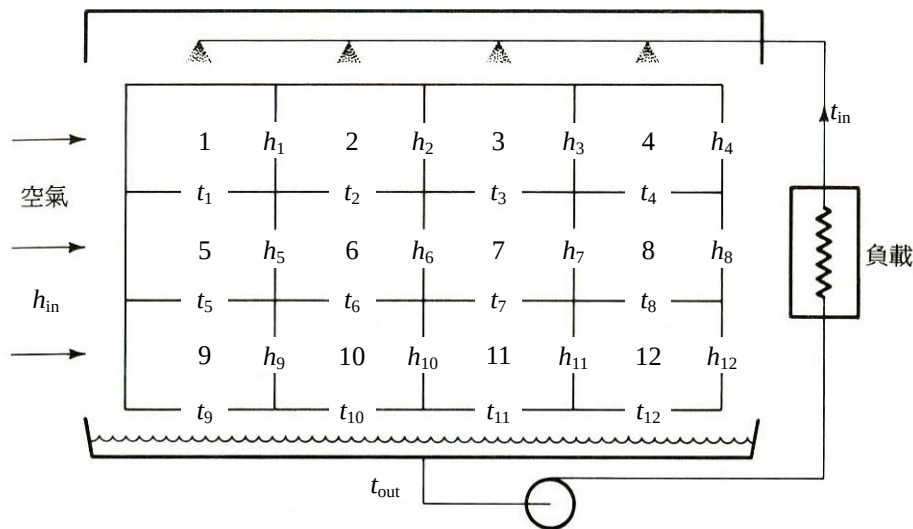
圖 1. 橫流式冷卻塔
