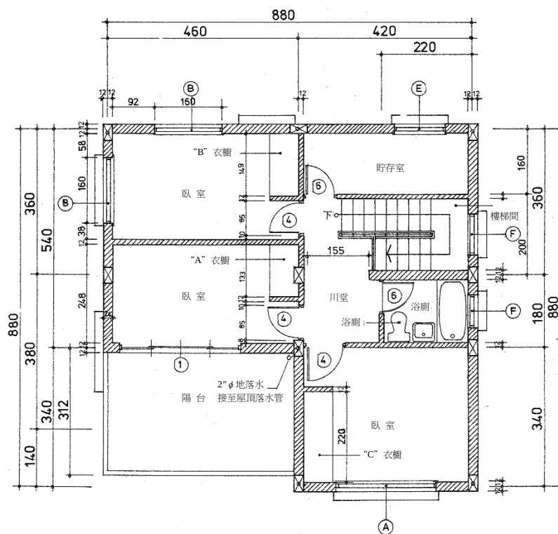
1B A-1 2樓平面圖 (單位：cm)
