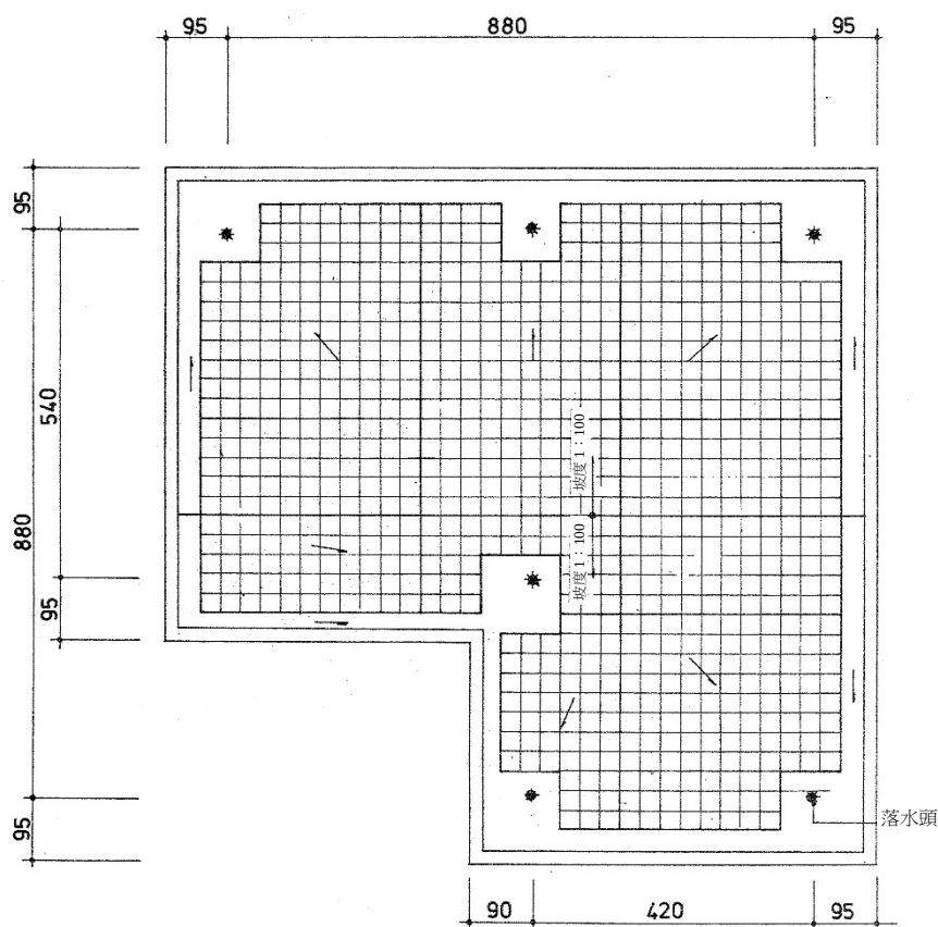
1A A-2 屋頂平面圖 (單位：cm)
