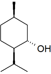
(+)-isomenthol
