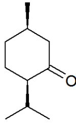
(+)-isomenthone
