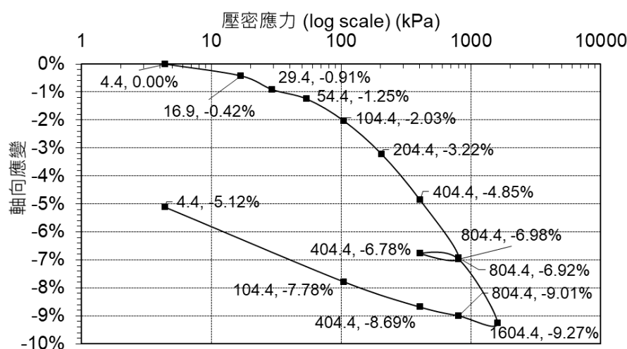
圖1 土壤壓密曲線
