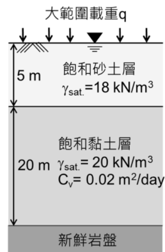
圖2 土層剖面
