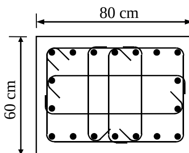
主筋18-D25
