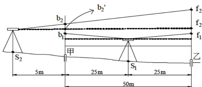
定樁(木樁)法校正法示意圖(未依比例)
