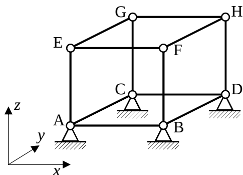
(a)三維空間桁架
