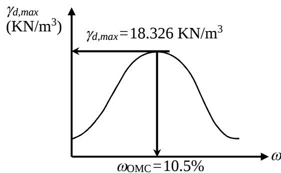
圖1. 填方土壤夯實曲線
