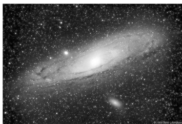
圖 23 仙女座大星系 M31
