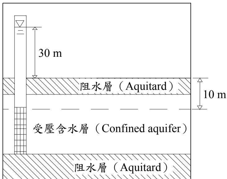
圖（A）受壓含水層示意圖
