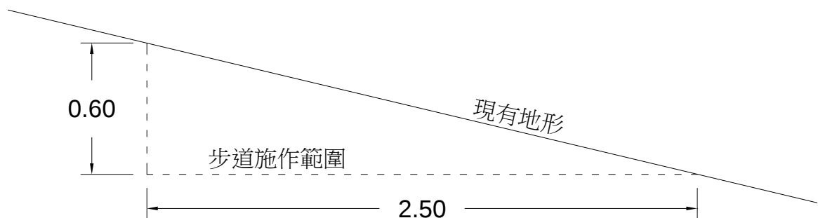
休憩步道施作剖面示意圖（單位：公尺）
